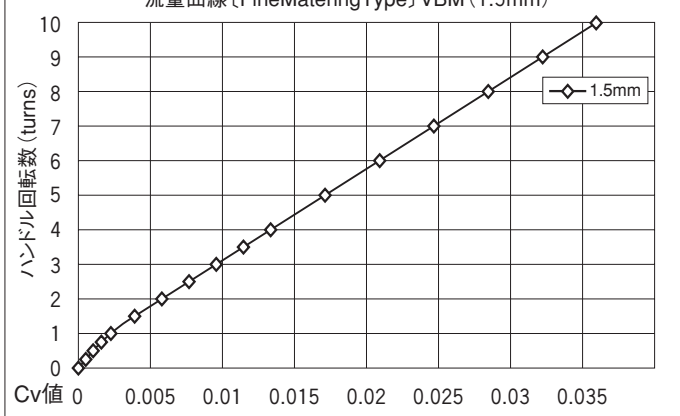
流量曲線 [FineMeteringType] VBM (1.5mm)
