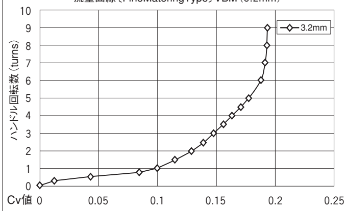
流量曲線 [FineMeteringType] VBM (3.2mm)
